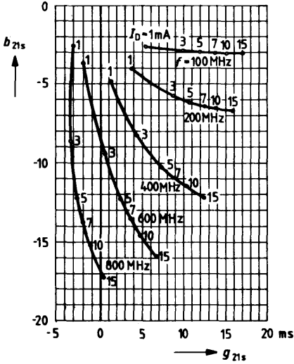
Gate 1 transmittance y_{21s} (source circuit); V_{DS} = 15\text{ V} ; mS V_{G2S} = 4\text{ V} ; I_{DSS} = 10\text{ mA}
