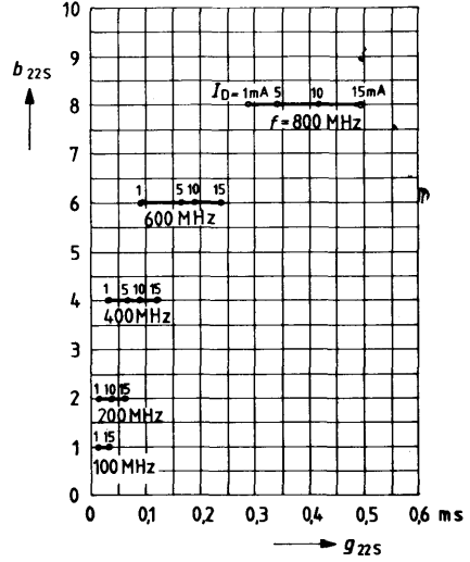
Output conductance y_{22s} (source circuit); V_{DS} = 15\text{ V} ; mS V_{G2} = 4\text{ V} ; I_{DSS} = 10\text{ mA}
