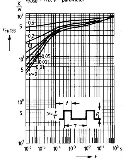
Permissible pulse load r_{thJSB} = f(t) ; \nu = parameter
